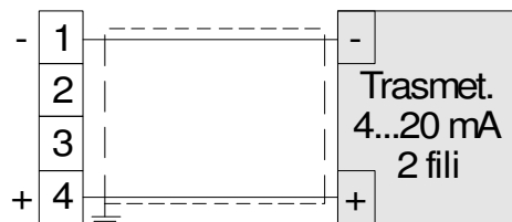
Fig. 8 Collegamento di segnali 0/4-20 mA a trasmettitore passivo con alimentazione ausiliaria
