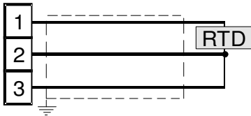
Fig. 5 Collegamento di termoresistenza
